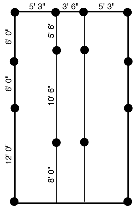
14 Ty-Down Standard
