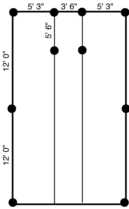
10 Ty-Down Standard
