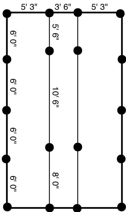
18 Ty-Down Standard
