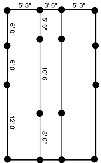
16 Ty-Down Standard
