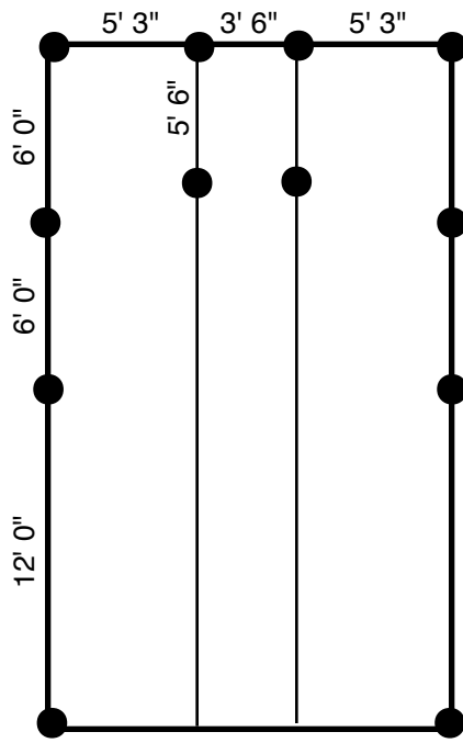
12 Ty-Down Standard
